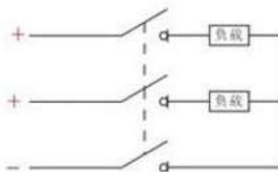
3层 (3P) 外形
